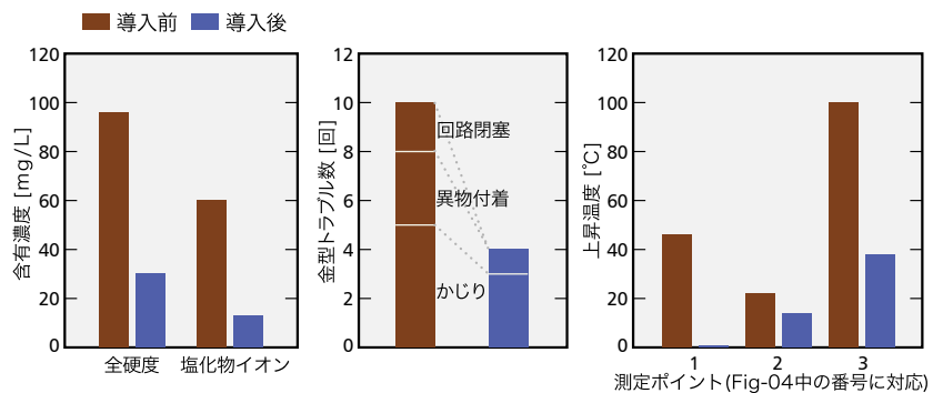
【Fig-06 二次冷却システム導入後の改善状況】
