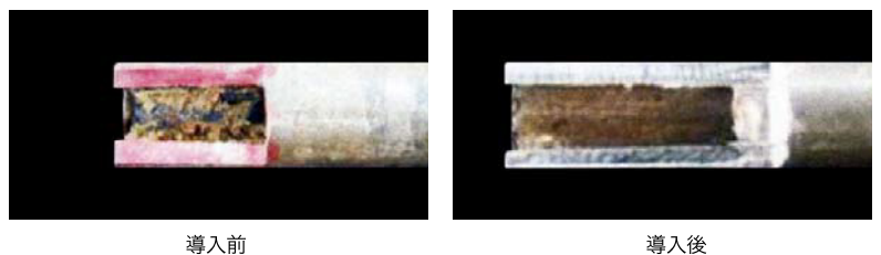
【Fig-07 冷却回路のスケールの比較】
